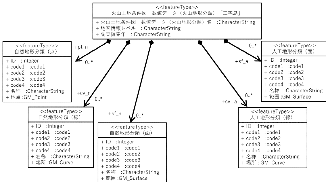
火山土地条件図 数値データ（火山地形分類）「三宅島」 応用スキーマ
