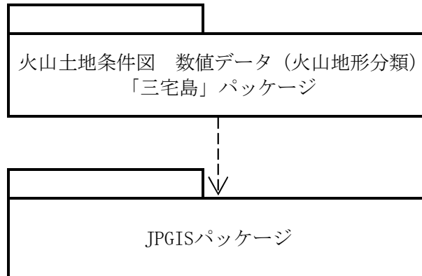
火山土地条件図 数値データ（火山地形分類）「三宅島」 応用スキーマパッケージ図
