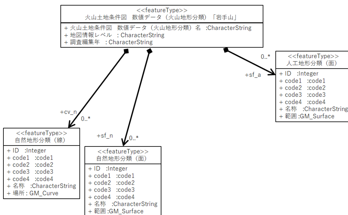
火山土地条件図 数値データ（火山地形分類）「岩手山」 応用スキーマ
