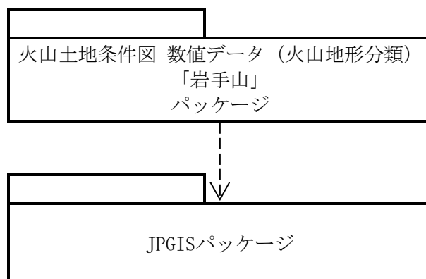
火山土地条件図 数値データ（火山地形分類）「岩手山」 応用スキーマパッケージ図
