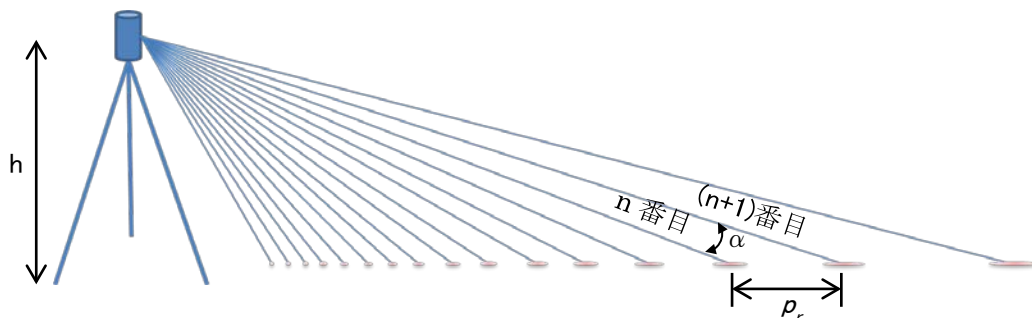
図 4 地上レーザースキャナによる観測状況立面図（水平な平坦面）
