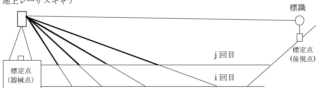
図 13 地形の変化観測のイメージ (—: i 回目、- -: j 回目)
