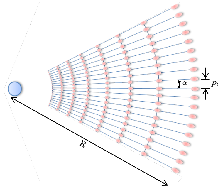
図 3 地上レーザースキャナによる観測状況平面図（水平な平坦面）
