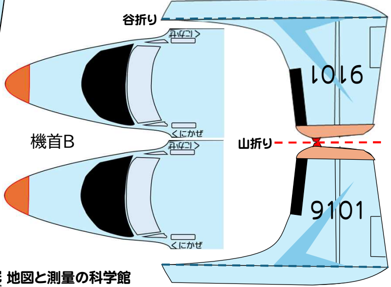
垂直尾翼
