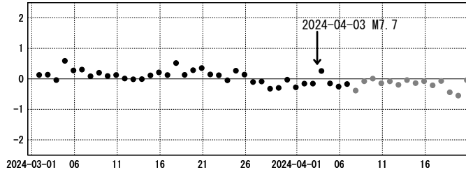
cm (2) 与論(950495)→波照間島(960751) 南北 基準値: -329070.615m
