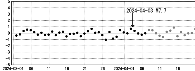
cm (2) 与論(950495)→波照間島(960751) 比高 基準値: -57.428m
