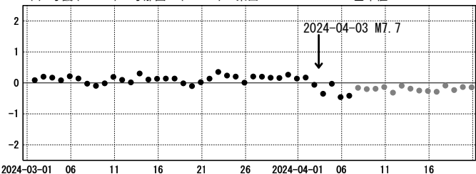
cm (1) 与論(950495)→与那国B(151211) 東西 基準値: -550574.001m
