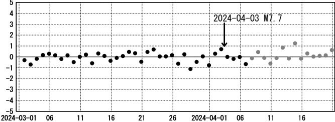
cm (1) 与論(950495)→与那国B(151211) 比高 基準値: -72.496m
