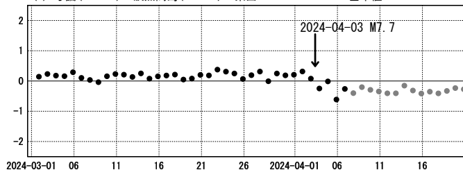
cm (2) 与論(950495)→波照間島(960751) 東西 基準値: -465833.694m
