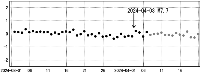
cm (1) 与論(950495)→与那国B(151211) 南北 基準値: -285589.750m
