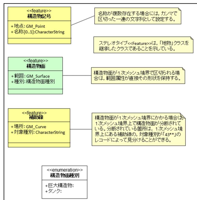
図 2-7 構造物サブパッケージ
