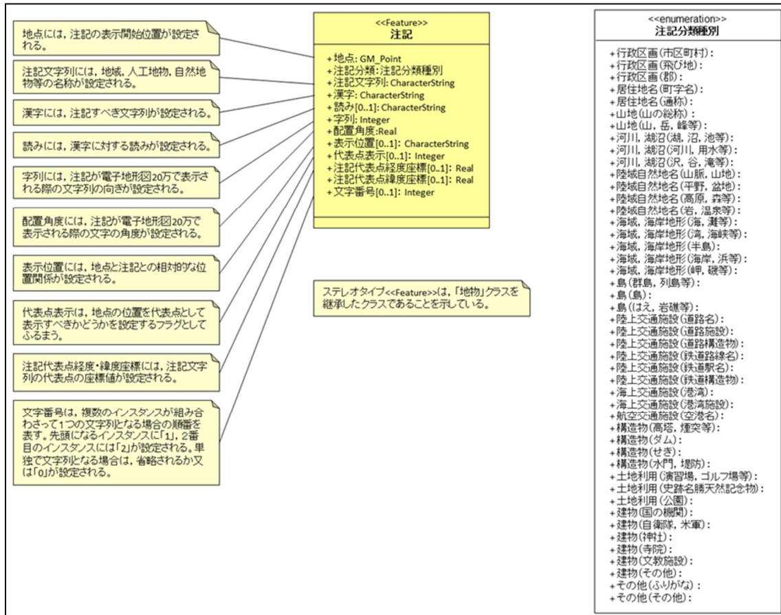
図 2-11 注記サブパッケージ
