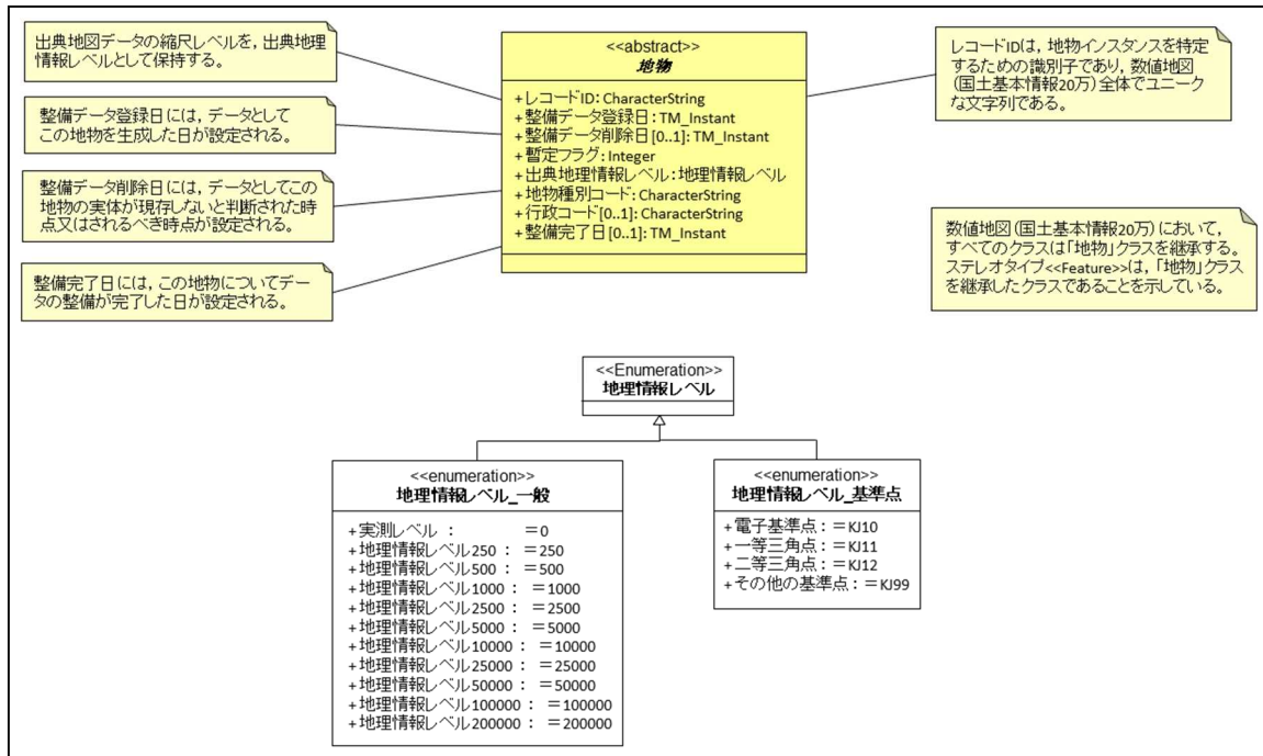
図 2-2 地物基本パッケージ
