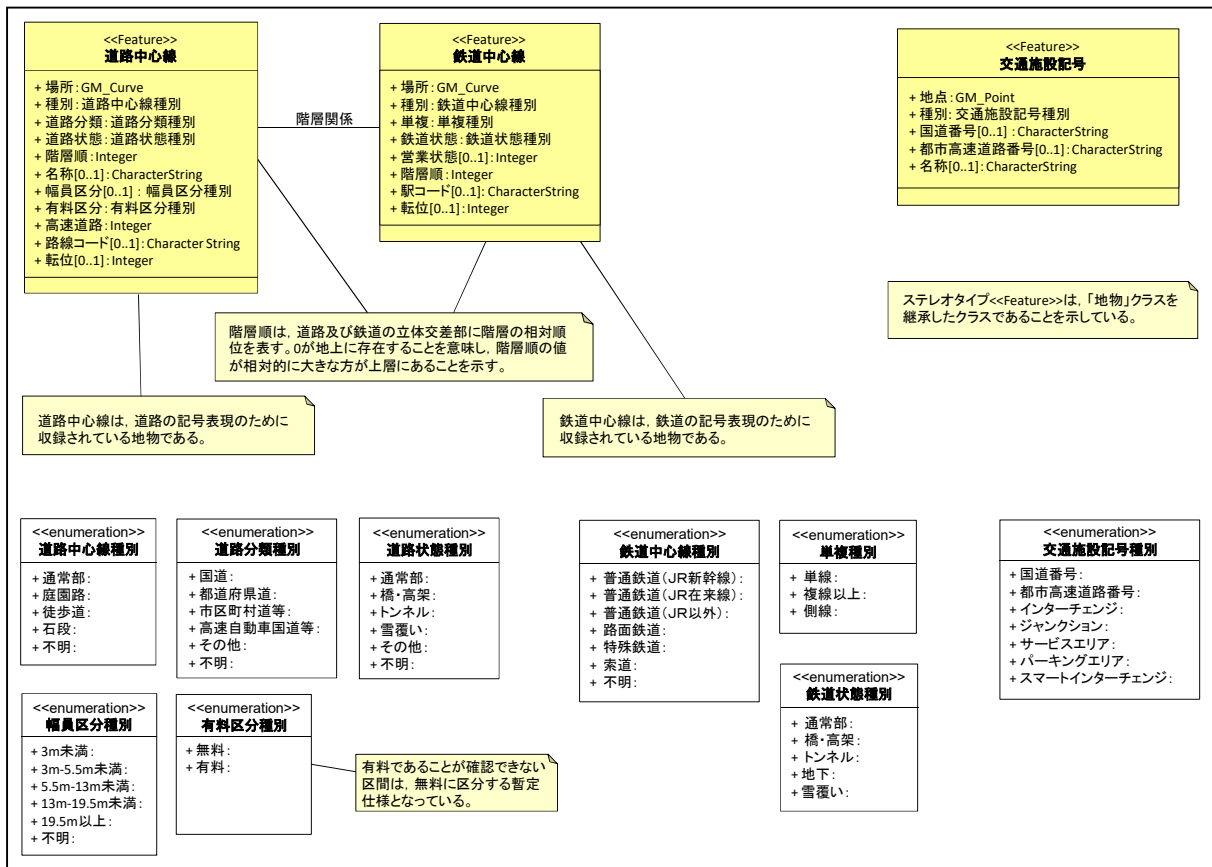
図 2-5 交通施設サブパッケージ
