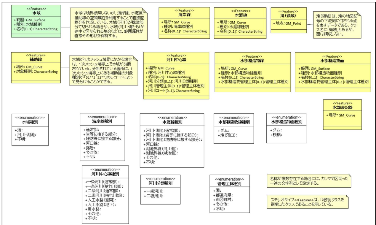
図 2-8 水部等サブパッケージ
