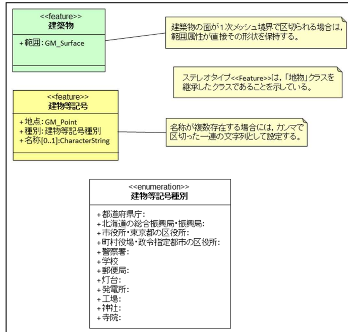
図 2-6 建物等サブパッケージ
