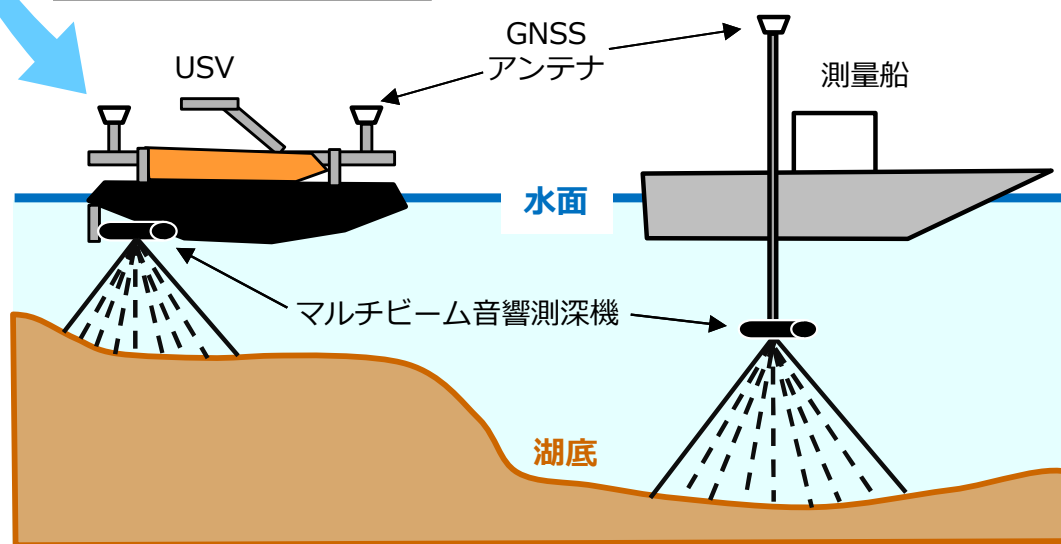
測量計画図のイメージ 小川原湖 (青森県)
