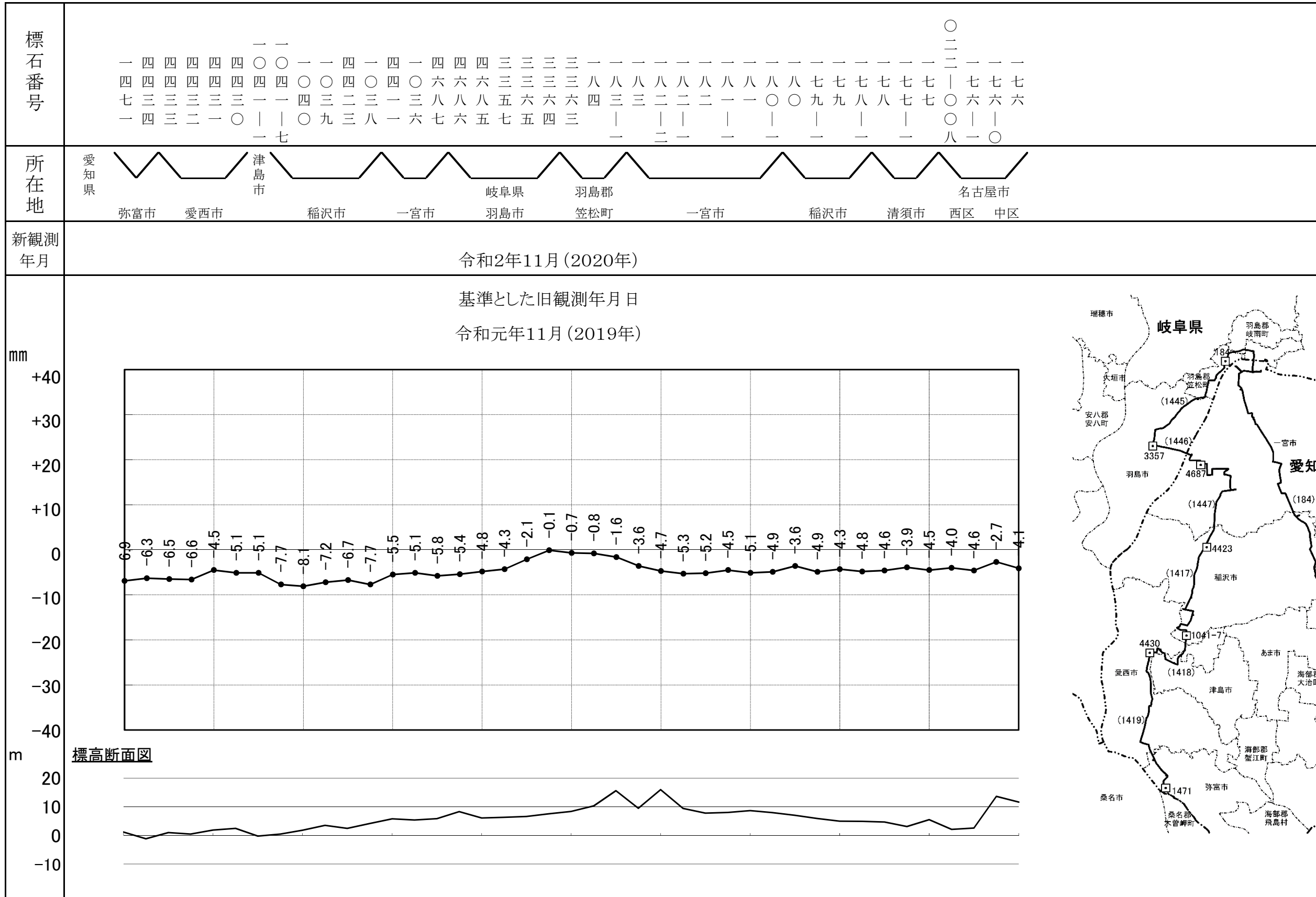
図5 - 2 基本水準点変動図
