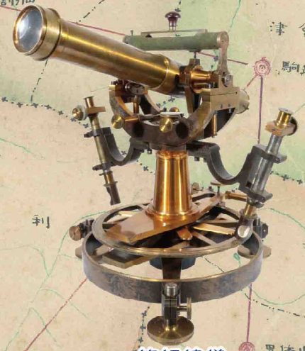
一等経緯儀 (カールツェッセル製：ドイツ)
