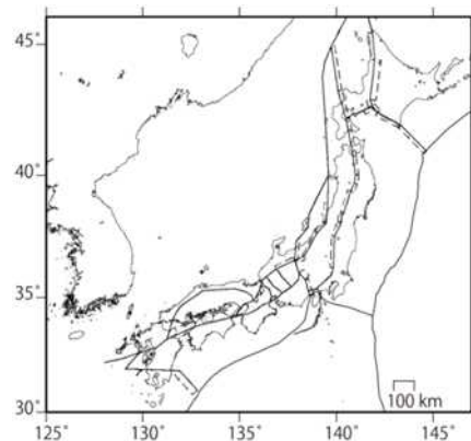
図-1 Loveless and Meade (2010) による日本列島のブロック断層モデル。
