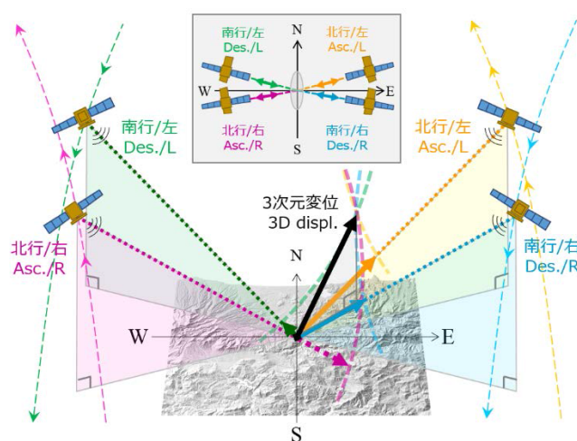
干渉 SAR 3次元解析の原理図
