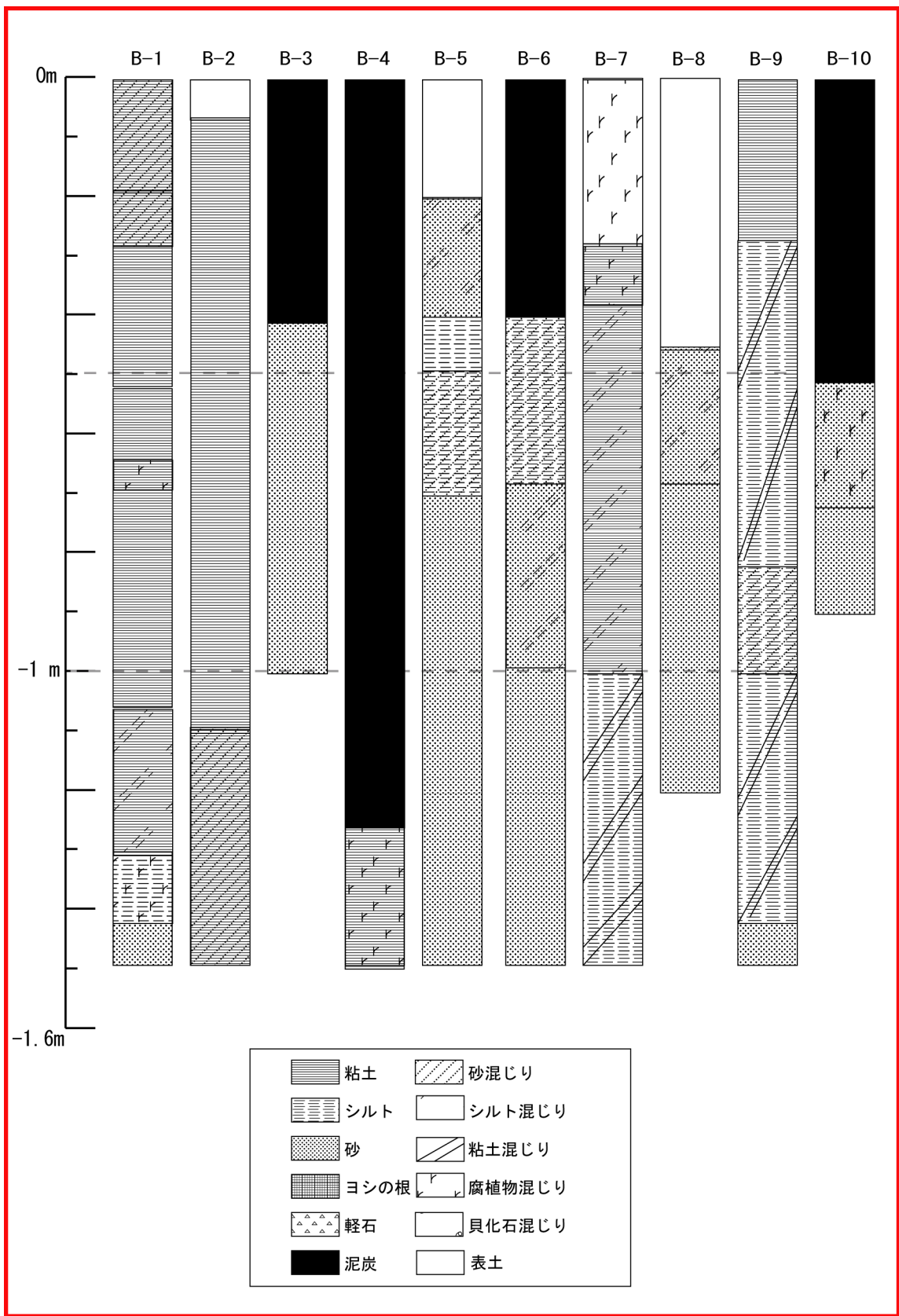
図 - 4 簡易ボーリング柱状図
