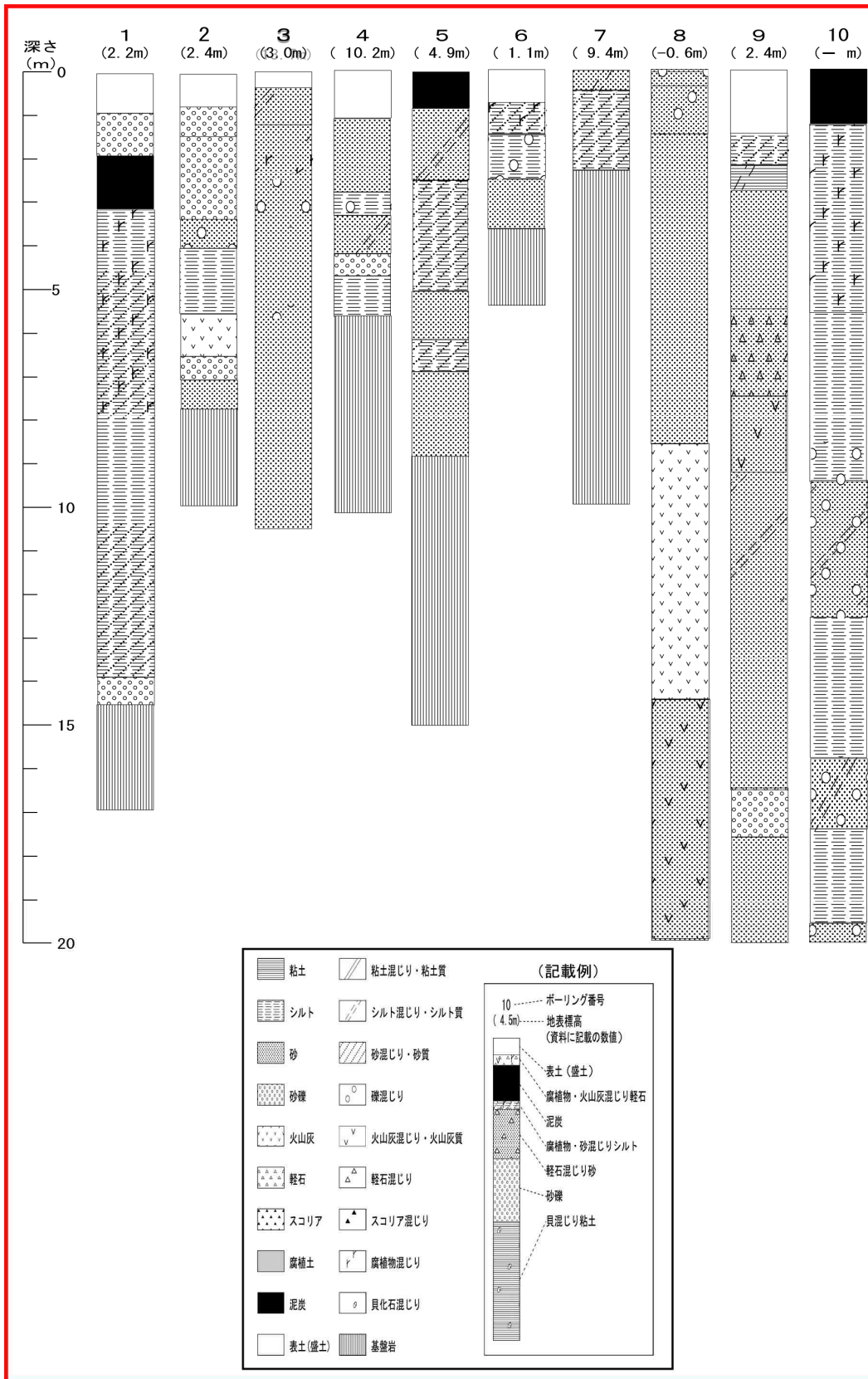
図 - 2 ボーリング柱状図
