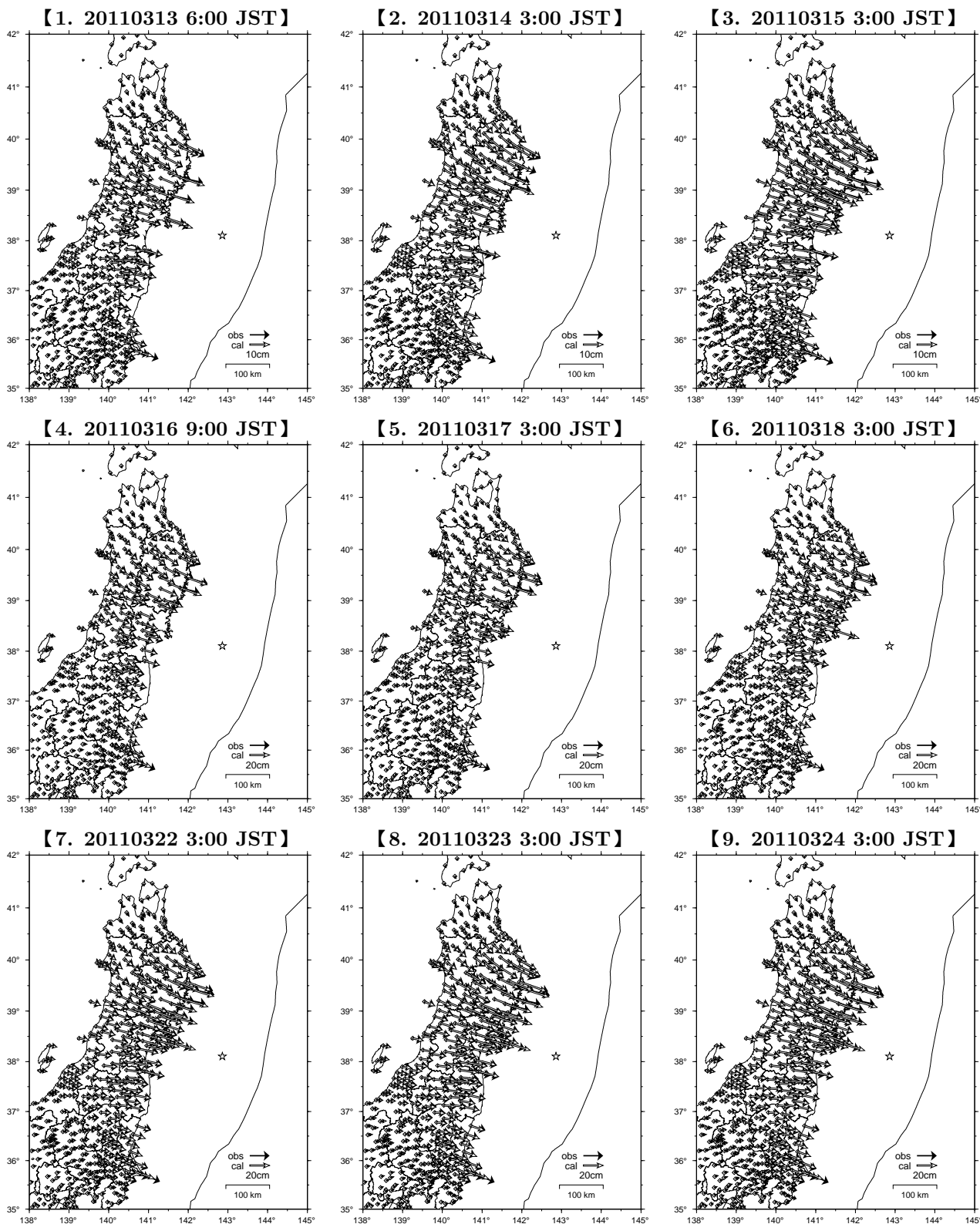
☆ : 本震の震央 ( 気象庁 ) . ☆ : Epicenter of the mainshock ( JMA ). 図 4 からスケールを変更している。 The scale is changed from panel 4.
