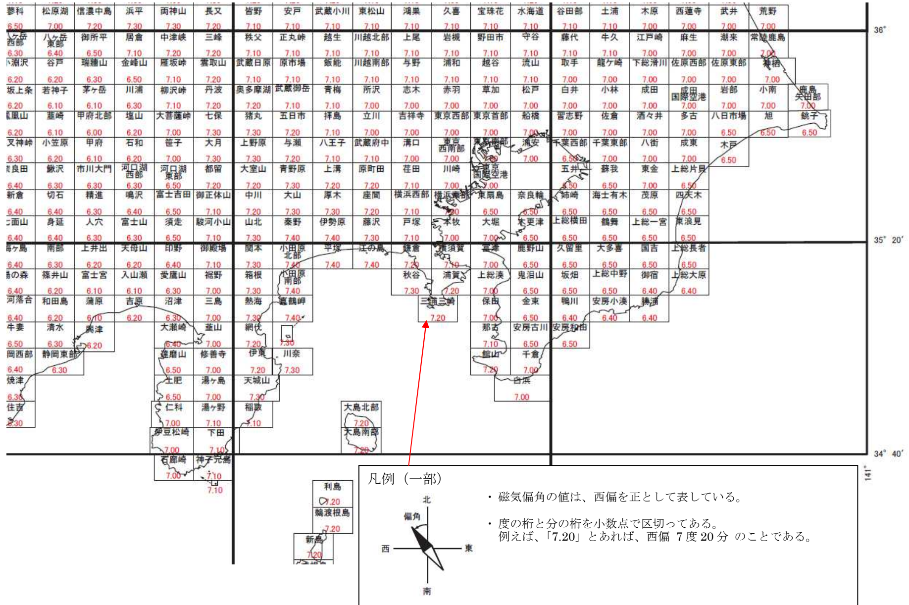
資料一 4 2010.0年値 磁気偏角一覽図（一部）
