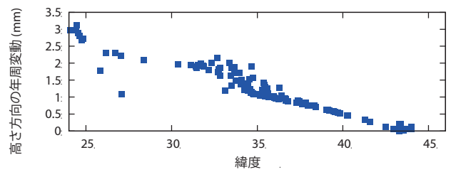
図-4 海洋荷重による電子基準点の高さの年周変動の振幅
