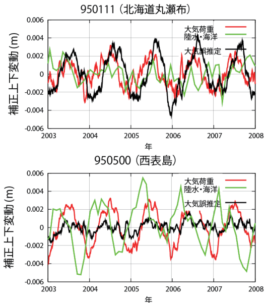
図-5 さまざまな誤差(変形)要因による電子基準点の高さの変動の例
