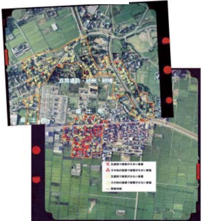
写真-15 砂押・柏木地区の建物被害
