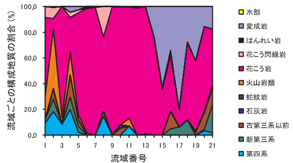
図-13 流域を構成する地質の割合。流域番号は表-2 と一致。
