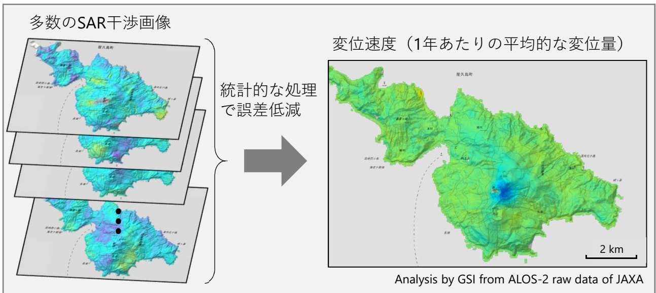
図1. 干渉SAR時系列解析の概要
