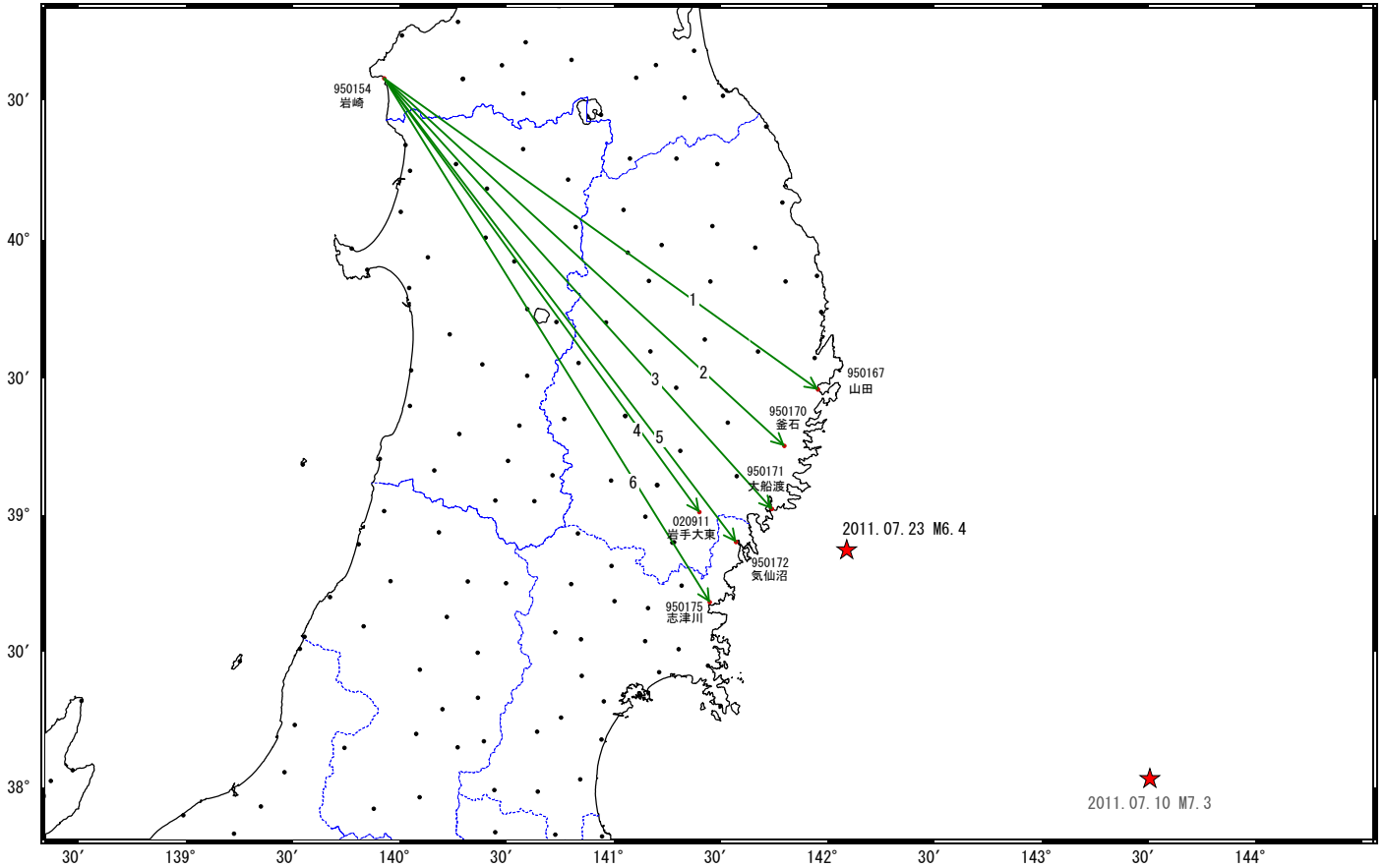
基線図
